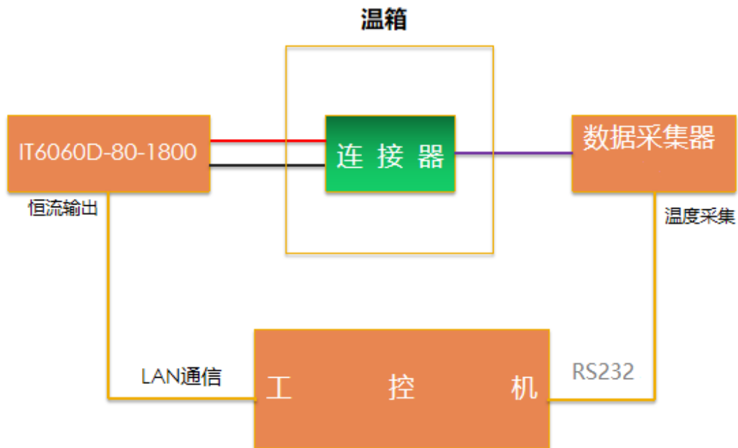
ITECH 温升测试系统原理图
